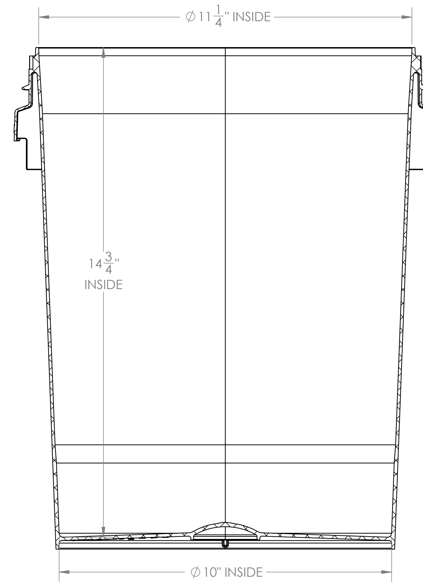
SECTION A-A
