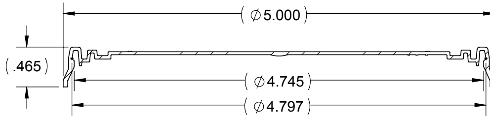
SECTION A-A SCALE 1 : 1
