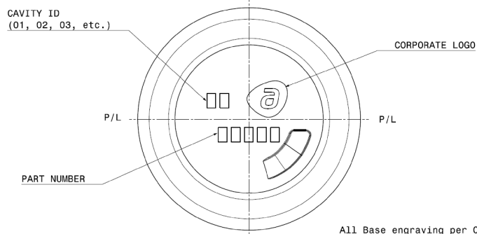
Bottom view Scale: 3:1
