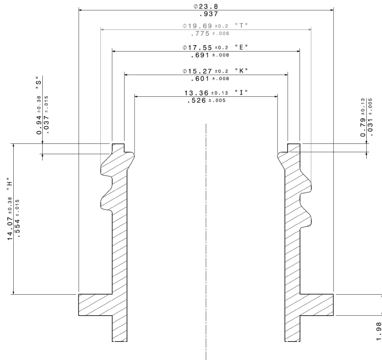
Section cut A-A Scale: 8:1
