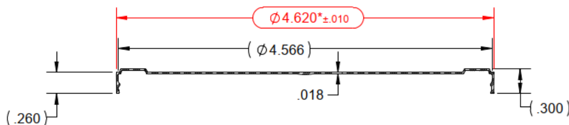
SECTION A-A SCALE 1 : 1
