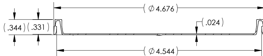
SECTION A-A SCALE 1 : 1
